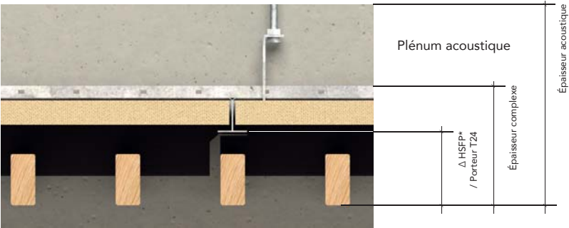
Détail
